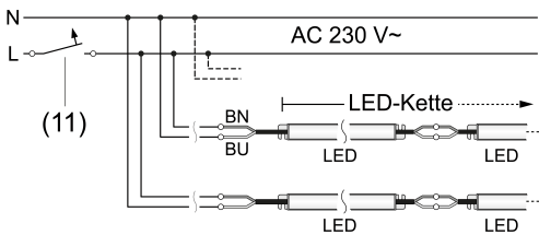
Bild 6: Schaltskizze
