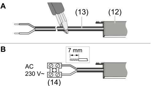
Bild 10: Ersten Lichteinsatz an Zuleitung anschließen (Sonderleuchte mit langer Eingangsleitung)
