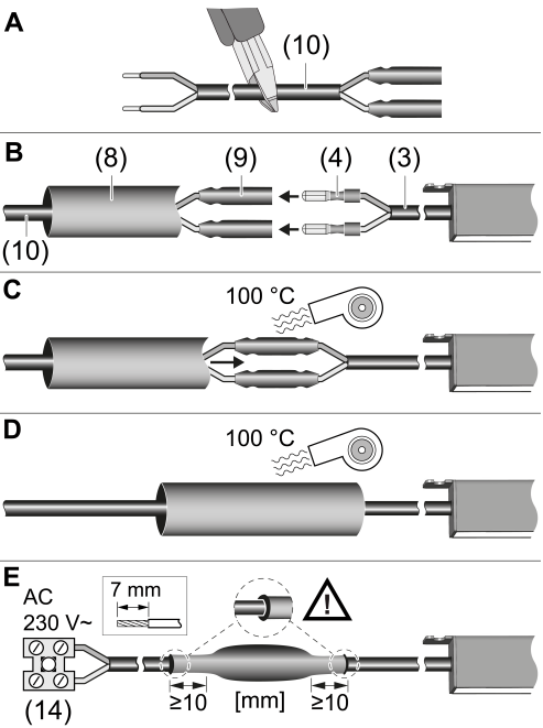
Bild 9: Ersten Lichteinsatz an Zuleitung anschließen (Standard-Leuchte mit Adapterkabel)
