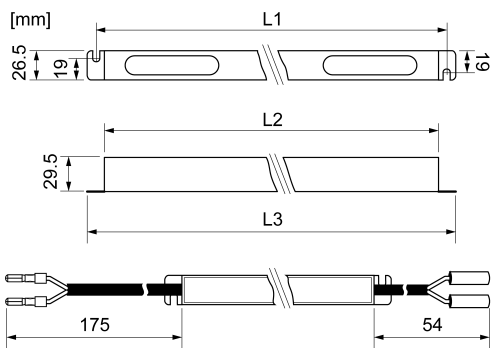
Bild 4: Maßzeichnung
