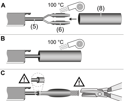
Bild 8: Ausgangsleitung des letzten Lichteinsatzes versiegeln
