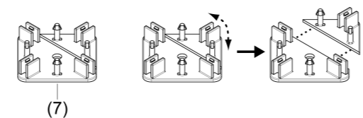
Bild 4: Verbinder teilen
