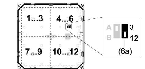
Bild 10: Anzahl Teilbereiche einstellen
