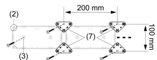
Bild 6: Montage mit Verbindern: LED-Lampe PR100
