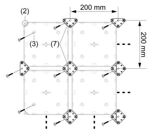
Bild 5: Montage mit Verbindern: LED-Lampe PQ200
