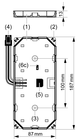
Bild 2: LED-Lampe PR100 (nur TW)
