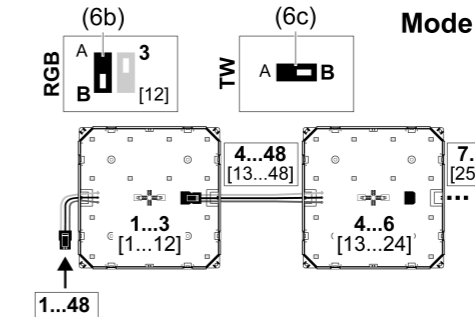
Bild 11: Modus für Adressierung einstellen
