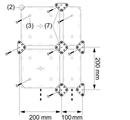
Bild 7: Montage mit Verbindern: LED-Lampe PQ200 und PR100 kombiniert
